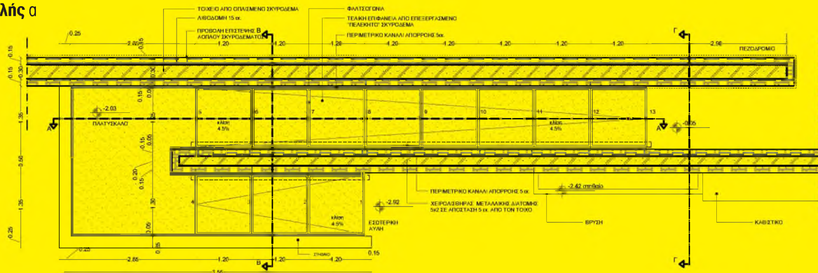
ΚΑΤΟΨΗ ΡΑΜΠΟΣΚΑΛΑΣ
